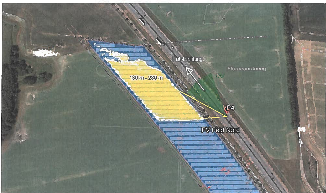
Bild 4.4.1: Simulation am Messpunkte P4 (Quelle: Google Earth/SolPEG)
