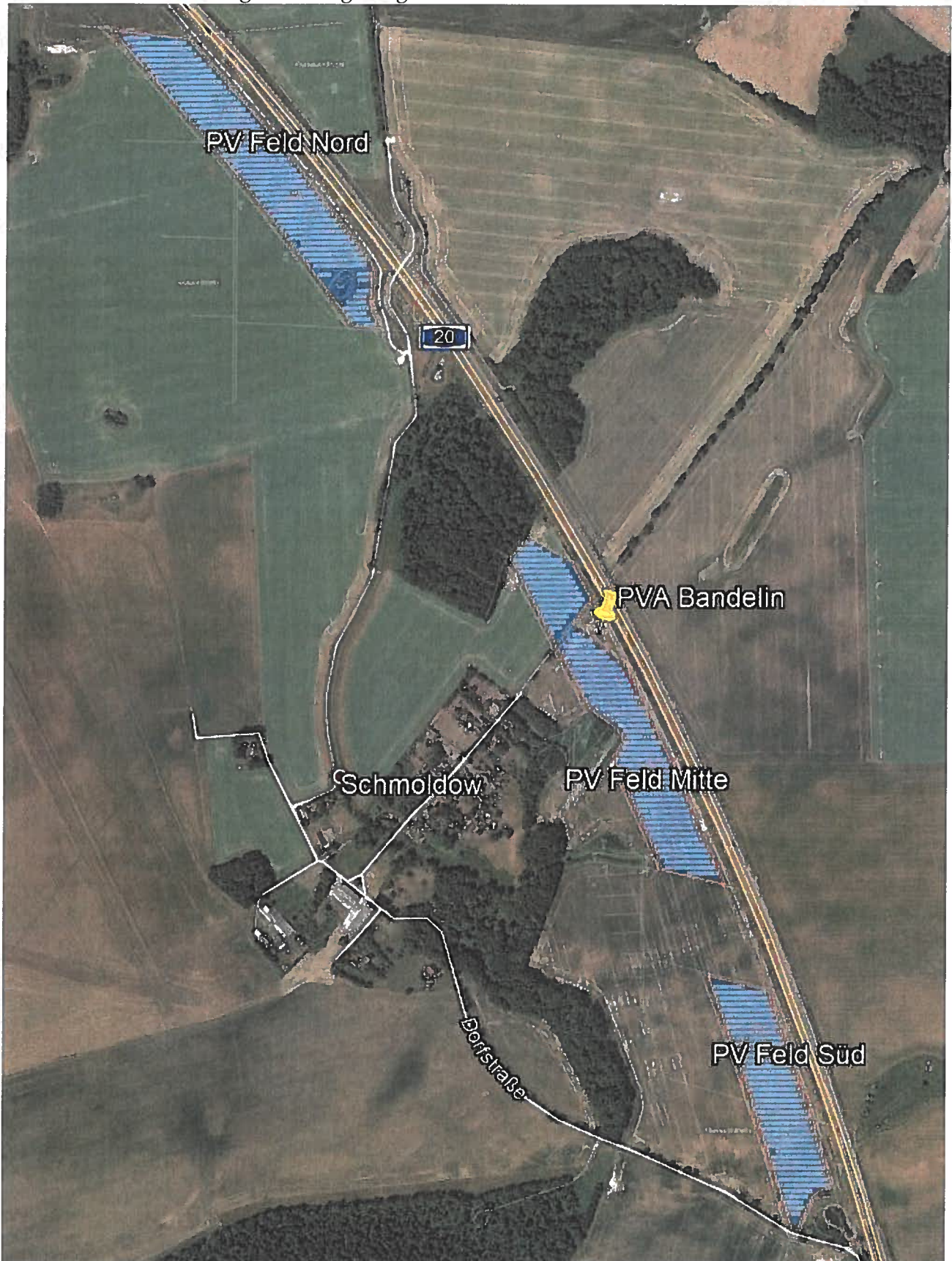
Bild 2.1.2: Detailansicht der PV Flächen (Quelle: Google Earth/SolPEG)
