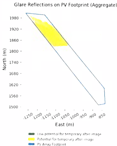
Bild 4.4.2: Ergebnisdetails für Messpunkt P4 (Quelle: Simulationsergebnisse)
