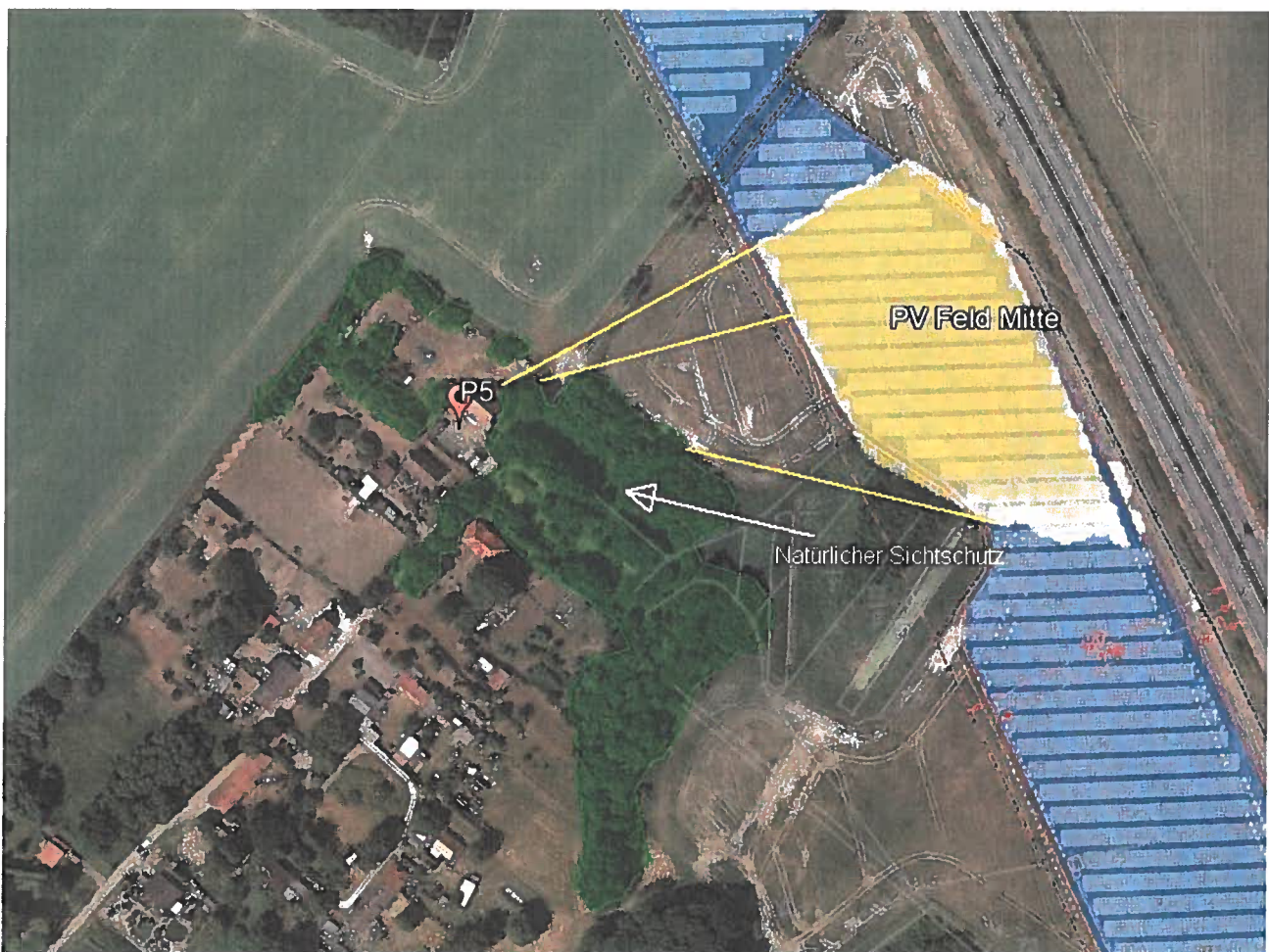
Bild 4.5.1: Simulation am Messpunkte P5 (Quelle: Google Earth/SolPEG)
