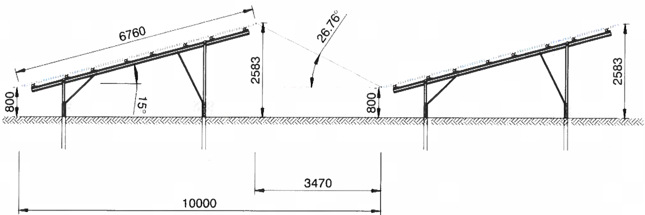
Bild 3.4.1: Skizzen der Modulkonstruktion (Quelle: Auftraggeber)
